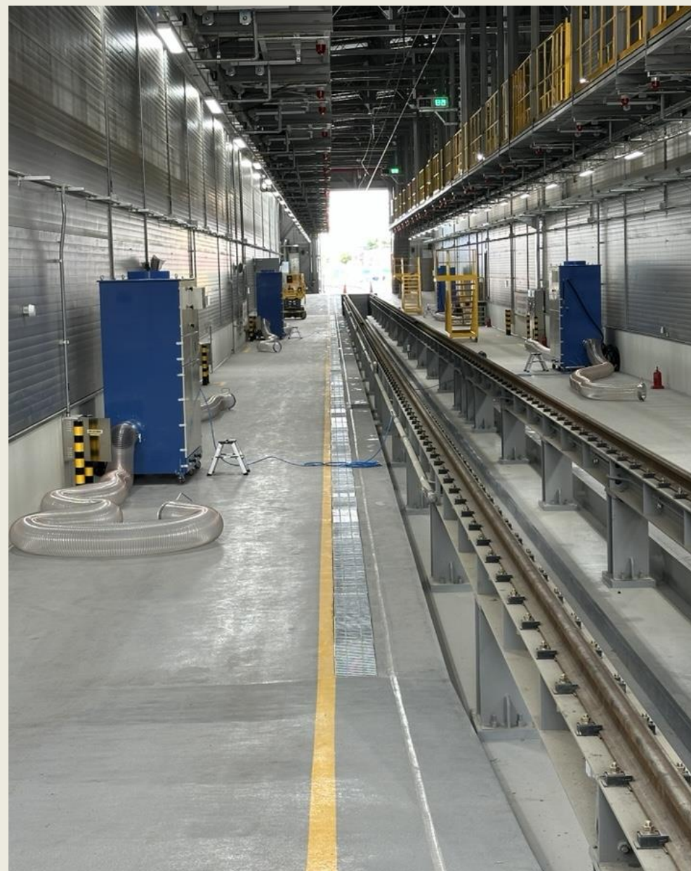
한국철도공사 대구기관차승무사업소 전동차 필터용 Air Pulse 집진기 (7,800 m 3 /hr-4 SET)
